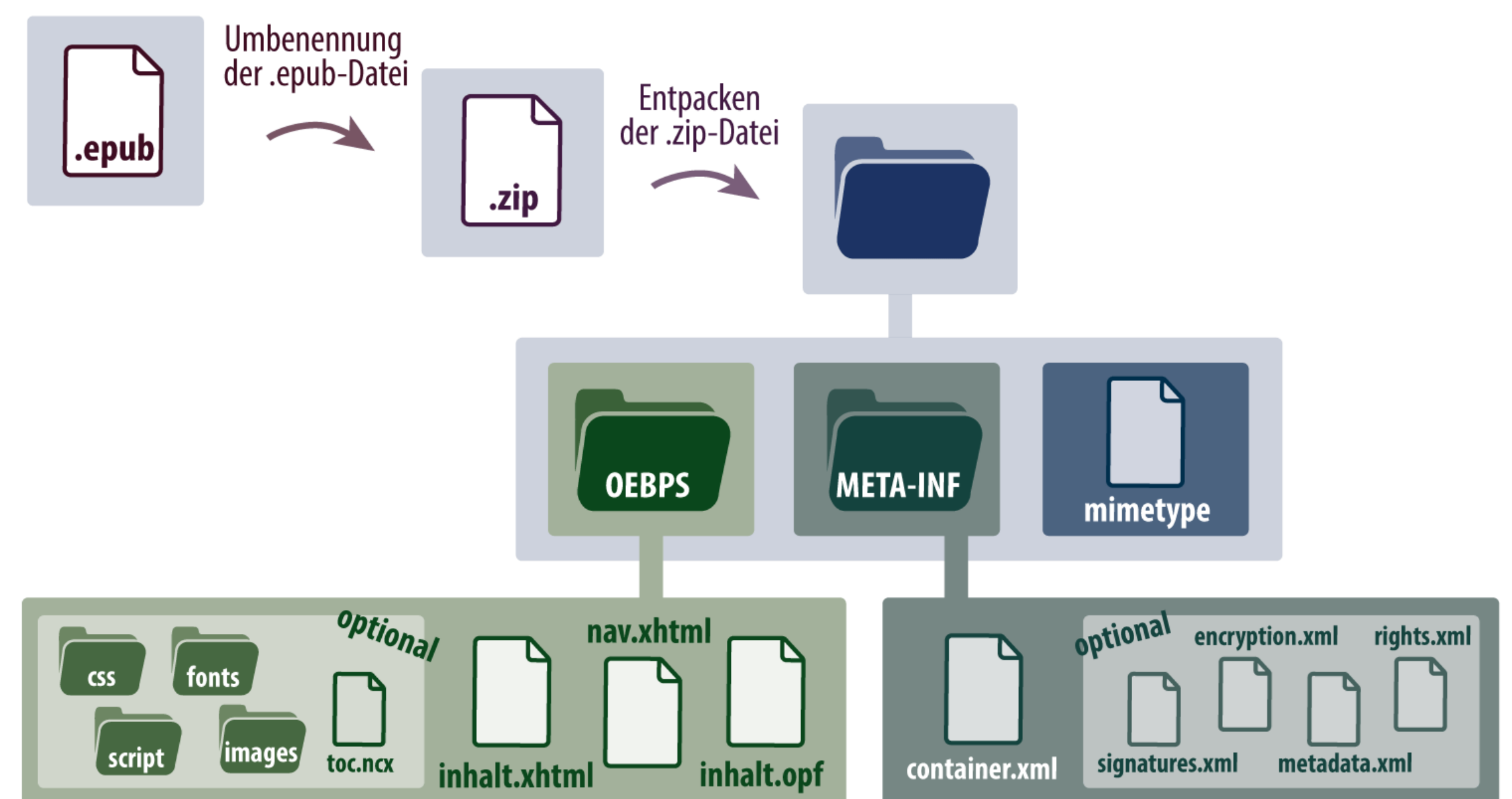
Struktur und Zugriff auf eine ePUB 3-Datei. Obligatorische und optionale Elemente
